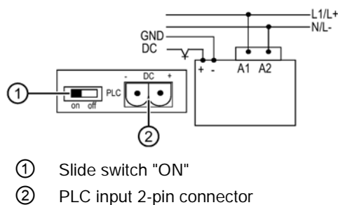
Figure 6-4 3RT1.6.-.N...-.... / 3RT1.7.-.N...-....
