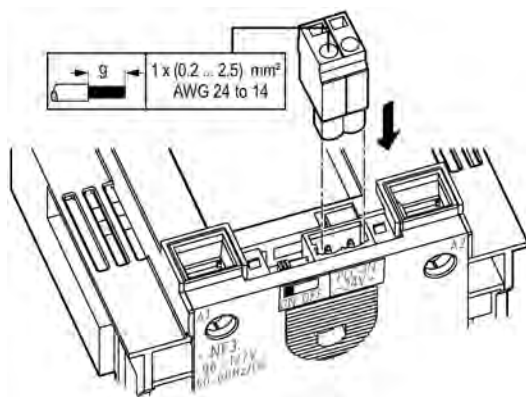
Figure 6-10 3RT1.6.-.X...-.... / 3RT1.7.-.X...-....
