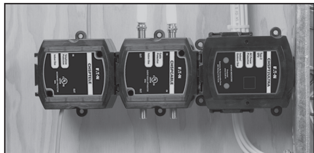
Figure 10. Joining CHSP Modules (3)/Jonction de modules CHSP (3)/Conexión de los módulos CHSP (3)
