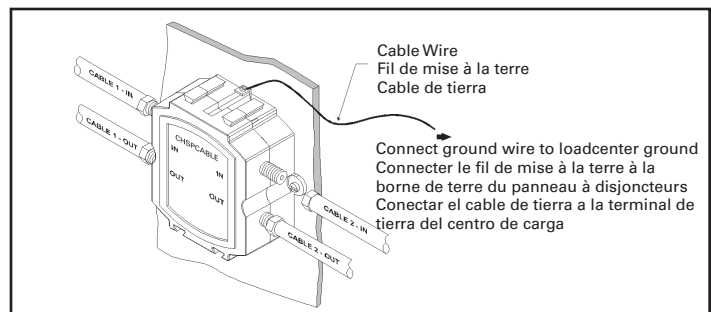
Figure 2. CHSPCABLE Wiring/Câblage du CHSPCABLE/Conexión de CHSPCABLE
